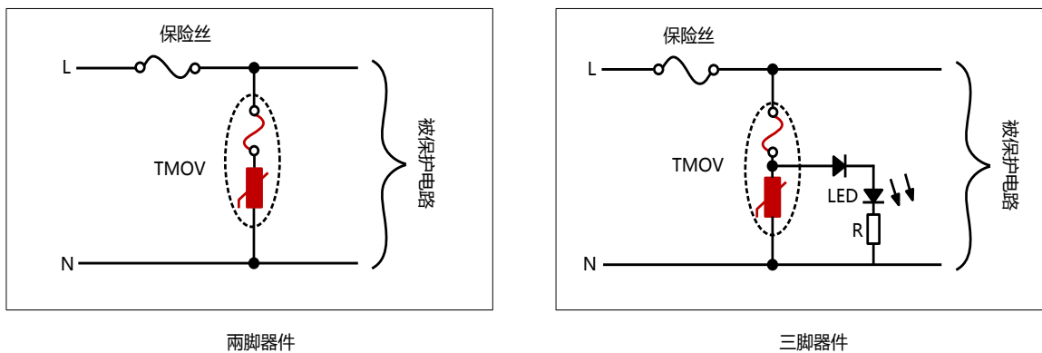
图 3 TMOV 应用连接图
