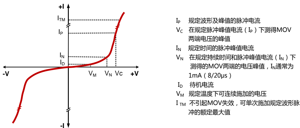
图 1 MOV 伏安特性曲线
