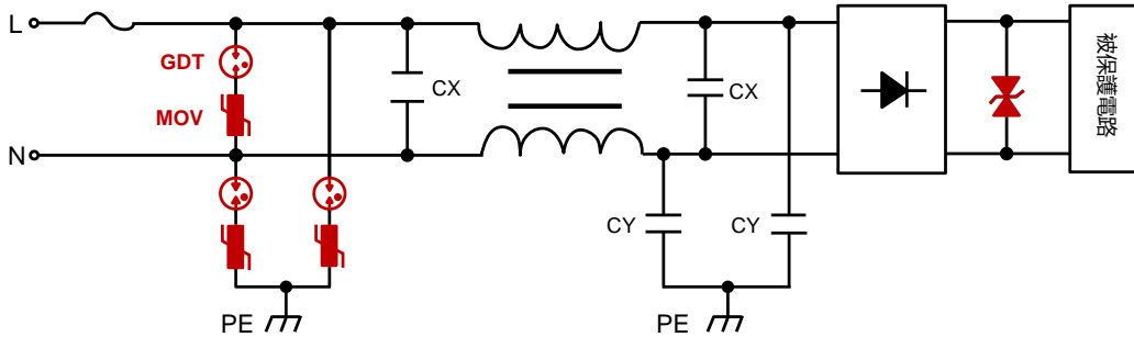
图 2 MOV 应用连接图
