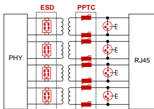
图 7 1000M RJ45 接口保护
