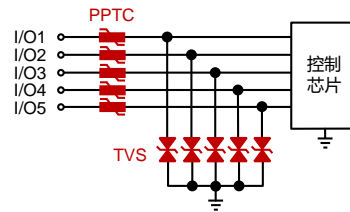
图 4 I/O 接口保护
