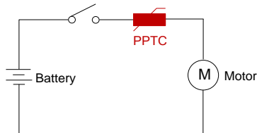
图 5 电机保护
